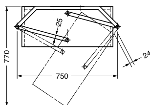
■キャビネット回転の寸法 (キャビネット幅680mmの場合)
